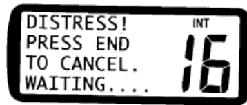
Chiamata Inviata
