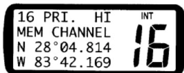
Visualizzazione Canale
