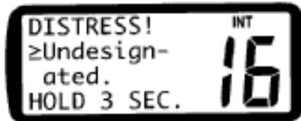
Schermo Allarme
