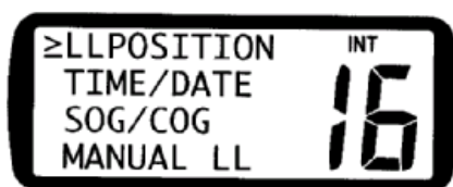
Selezione Data
