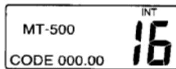
Schermo
