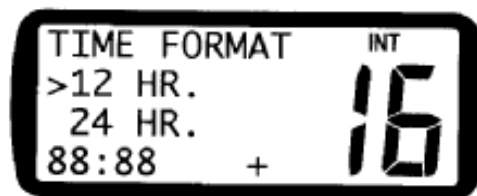
Selezione Formato
