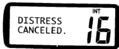
Chiamata Annullata
