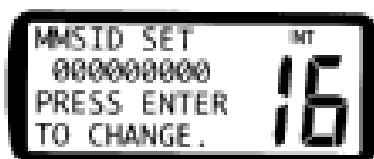
Impostazione MMSID
