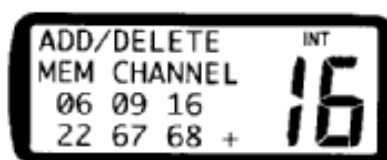
Lista Memoria
