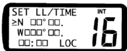
Registrazione Manuale
